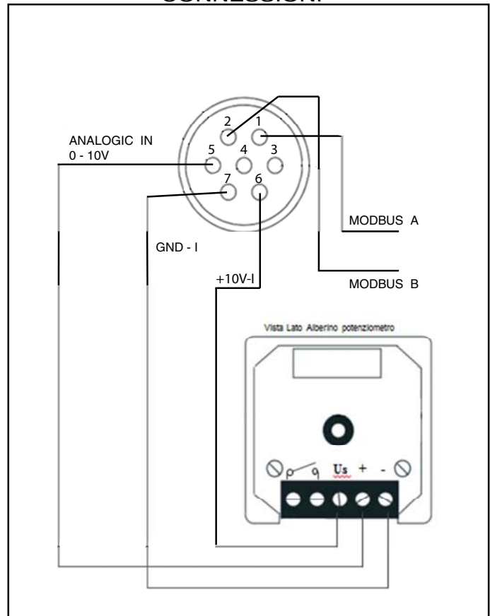
DETTAGLIO CONNESSIONI
